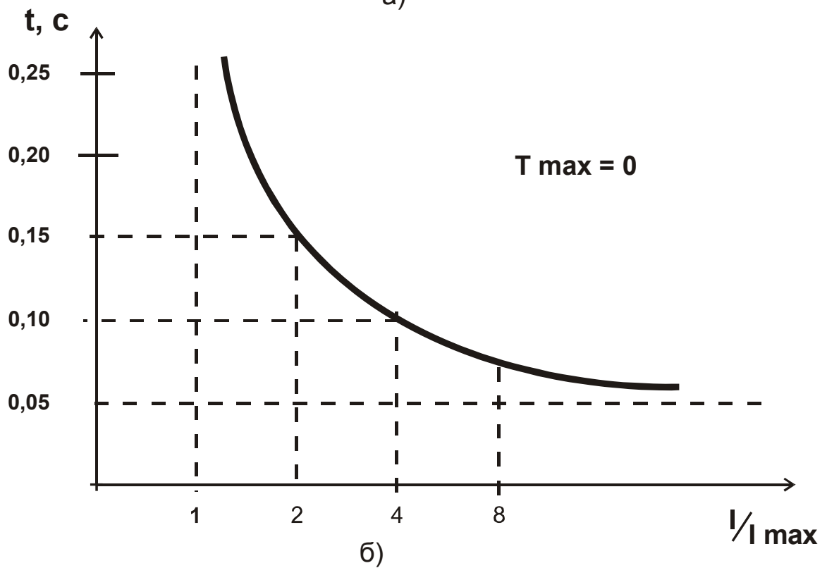
Рисунок 6 - характеристика защитного отключения контроллера
