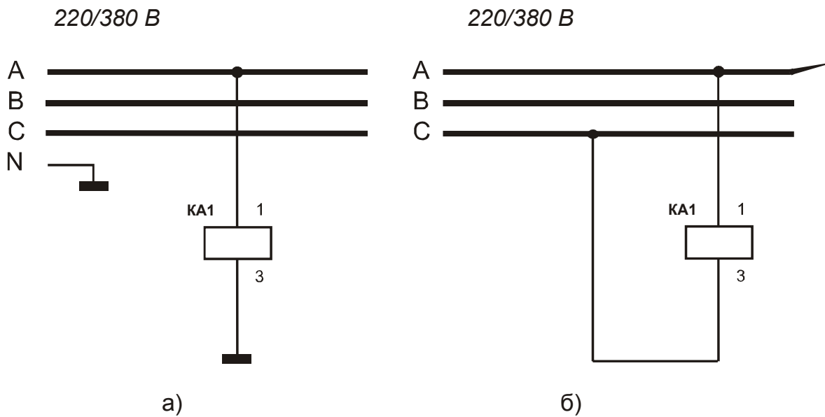
Рисунок 3 - схема питания контроллера от источника переменного напряжения 220 В (а) или 380 В (б).
