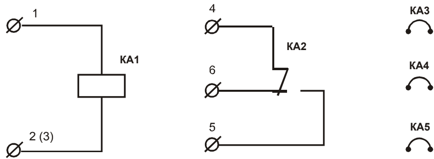
Рисунок 2 -условное графическое обозначение контроллера.
